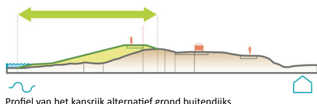
Profiel van het kansrijk alternatief grond buitendijks
