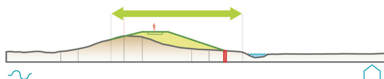
Profiel van het kansrijk alternatief constructie met grond binnendijks
