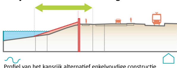
Profiel van het kansrijk alternatief enkelvoudige constructie
