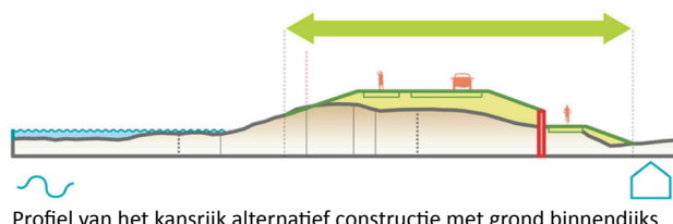
Profiel van het kansrijk alternatief constructie met grond binnendijks
