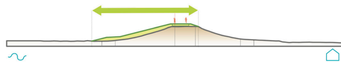
Profiel van het kansrijk alternatief grond buitendijks
