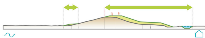
Profiel van het kansrijk alternatief grond binnendijks
