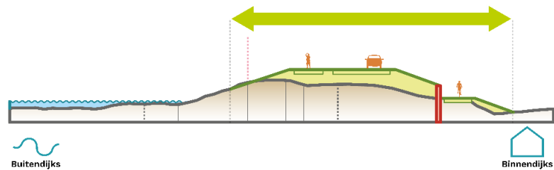
Constructie met grond
