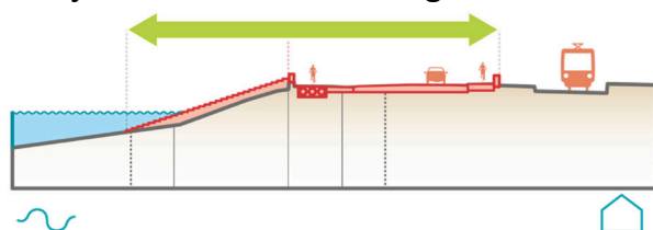
Profiel van het kansrijk alternatief meervoudige constructie
